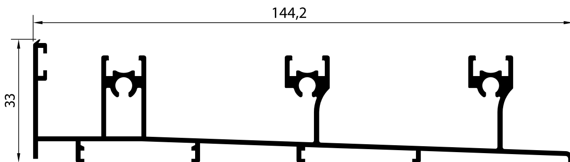
35150 (1446 gr/m) ΤΡΙΠΛΟΣ ΟΔΗΓΟΣ TRIPLE SASH FRAME
