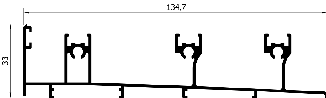
35138 (1388 gr/m) ΟΔΗΓΟΣ (ΕΠΑΛΛΗΛΟ-ΣΗΤΑ) RUNNING SASH FRAME (GLASS-SCREEN)
