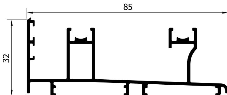
35182 (912 gr/m) ΟΔΗΓΟΣ ΧΩΝΕΥΤΟΣ (ΤΖΑΜΙ-ΠΑΤΖΟΥΡΙ 85 mm) SASH FRAME INWALL (GLASS-SHUTTER 85 mm)
