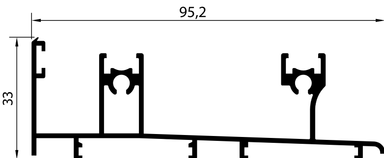
35140 (1018 gr/m) ΔΙΠΛΟΣ ΟΔΗΓΟΣ DOUBLE SASH FRAME
