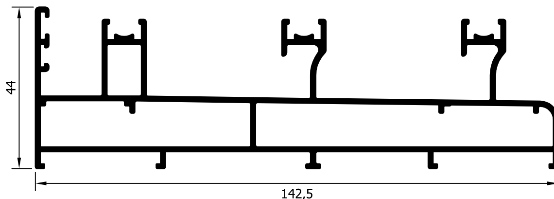
35183 (1940 gr/m) ΤΡΙΠΛΟΣ ΟΔΗΓΟΣ ΣΩΛΗΝΩΤΟΣ TRIPLE TUBED SASH FRAME
