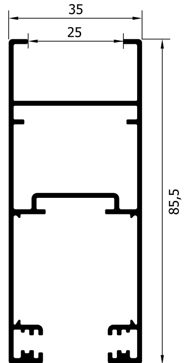
35224 (1117 gr/m) ΦΥΛΛΟ ΤΖΑΜΙΟΥ- ΠΑΤΖΟΥΡΙΟΥ ΙΣΙΟ WING (GLASS-SHUTTER) FLAT
