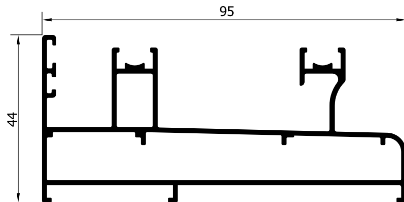
35180 (1345 gr/m) ΟΔΗΓΟΣ ΕΠΑΛΛΗΛΟΥ ΣΩΛΗΝΩΤΟΣ TUBED OVERLAPING SASH FRAME
