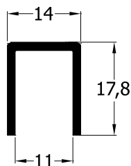
22028 (176 gr/m) ΠΡΟΣΘΗΚΗ ΦΥΛΛΟΥ 35215-35224 ΓΙΑ ΚΛΕΙΔΑΡΙΑ IN LINE ADAPTOR FOR IN LINE LOCK
