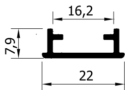
22025 (162 gr/m) ΠΡΟΣΘΗΚΗ ΦΥΛΛΟΥ 35219 ΓΙΑ ΚΛΕΙΔΑΡΙΑ IN LINE IN LINE ADAPTOR
