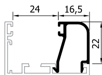
22216 (247 gr/m) ΚΑΜΠΥΛΩΤΟ ΠΗΧΑΚΙ ROUND GLAZING BEAD
