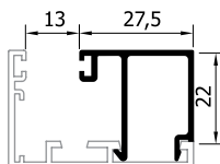
22131 (308 gr/m) ΙΣΙΟ ΠΗΧΑΚΙ SQUARE GLAZING BEAD
