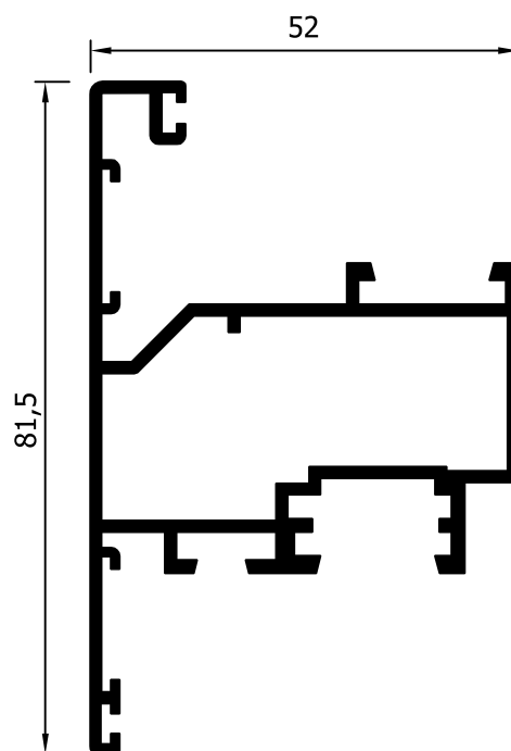
52225 (1095 gr/m) ΙΣΙΟ ΦΥΛΛΟ ΠΕΡΙΣΤΡΕΦΟΜΕΝΟ FLAT WING ON PIVOTS
