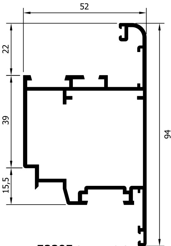
52205 (1210 gr/m) ΦΥΛΛΟ ΜΕΓΑΛΟ ΕΞΩΤ. ΑΝΟΙΓΟΜΕΝΟ BIG WING OUTSIDE OPENING
