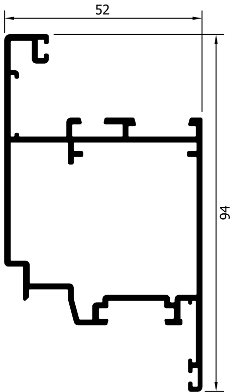
52220 (1218 gr/m) ΦΥΛΛΟ ΠΟΡΤΑΣ ΙΣΙΟ DOOR WING
