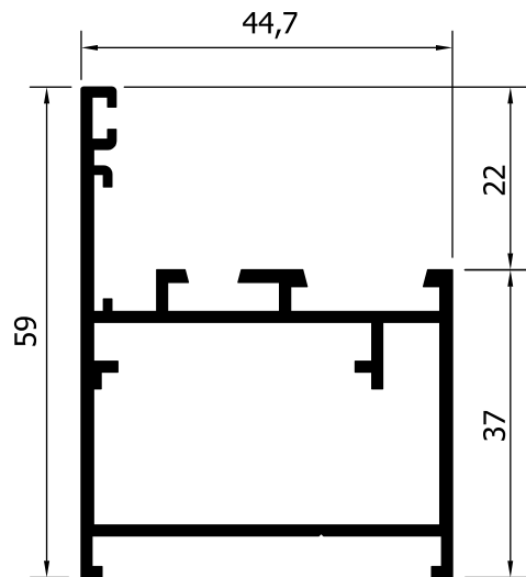
52107 (851 gr/m) ΚΑΣΑ ΙΣΙΑ FLAT FRAME
