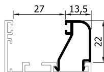
22501 (242 gr/m) ΚΑΜΠΥΛΩΤΟ ΠΗΧΑΚΙ ROUND GLAZING BEAD
