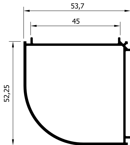
52102 (628 gr/m) ΓΩΝΙΑΚΗ ΚΟΛΩΝΑ 90° COLUMN FOR ANGLE 90°
