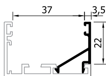
22133 (171 gr/m) ΙΣΙΟ ΠΗΧΑΚΙ SQUARE GLAZING BEAD
