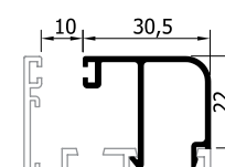
22230 (310 gr/m) ΚΑΜΠΥΛΩΤΟ ΠΗΧΑΚΙ ROUND GLAZING BEAD
