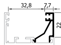
22132 (227 gr/m) ΙΣΙΟ ΠΗΧΑΚΙ SQUARE GLAZING BEAD
