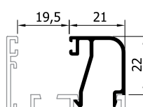
22221 (269 gr/m) ΚΑΜΠΥΛΩΤΟ ΠΗΧΑΚΙ ROUND GLAZING BEAD
