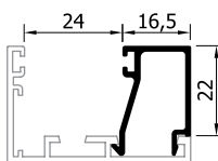
22129 (255 gr/m) ΙΣΙΟ ΠΗΧΑΚΙ SQUARE GLAZING BEAD
