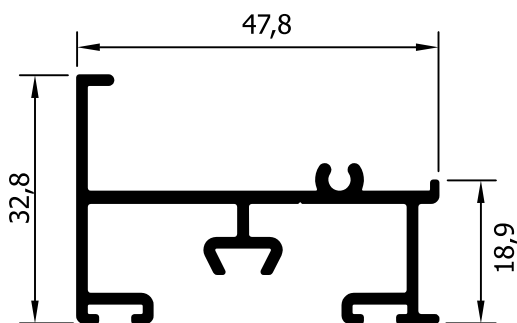
52319 (581 gr/m) ΠΡΟΣΘΗΚΗ ΣΤΕΓΑΝΩΣΗΣ ΠΟΡΤΑΣ ADDITIONAL PROFILE ON SEALING DOOR
