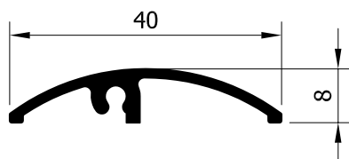
22008 (227 gr/m) ΚΑΤΩΚΑΣΙ ΓΙΑ ΠΟΡΤΕΣ THRESHOLD
