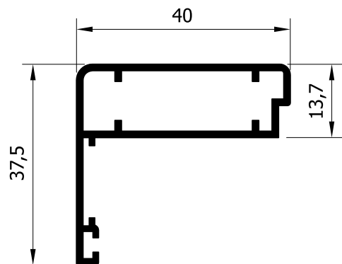
52129 (461 gr/m) ΠΡΟΣΘ.ΚΑΣΑ ΑΡΜΟΚΑΛ. (ΣΥΝΕΡΓ. ΜΕ 52128) ADDITIONAL SLIDING FRAME (COMBINED WITH 52128)
