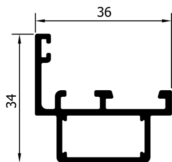
52321 (517 gr/m) ΚΑΣΑ ΓΙΑ ΚΑΙΤΙ ΜΕ ΠΗΧΑΚΙ (γωνία σύνδεσης E - 0423) FRAME DIVIDER WITH BEAD FOR CONNECTING CORNER E - 0423
