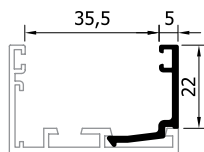
22134 (207 gr/m) ΙΣΙΟ ΠΗΧΑΚΙ SQUARE GLAZING BEAD
