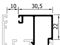
22130 (318 gr/m) ΙΣΙΟ ΠΗΧΑΚΙ SQUARE GLAZING BEAD
