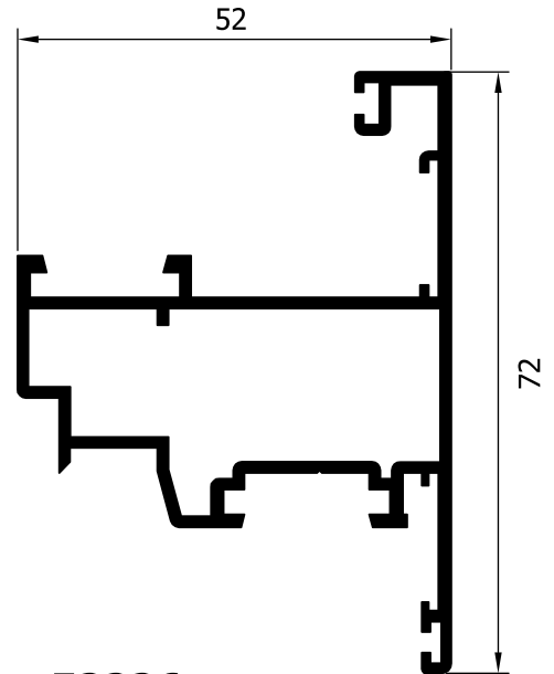
52226 (973 gr/m) ΙΣΙΟ ΦΥΛΛΟ ΕΞΩΤ. ΑΝΟΙΓΟΜΕΝΟ FLAT WING OPENING OUTSIDE
