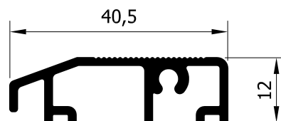
22020 (370 gr/m) ΚΑΤΩΚΑΣΙ ΠΟΡΤΑΣ DOOR THRESHOLD
