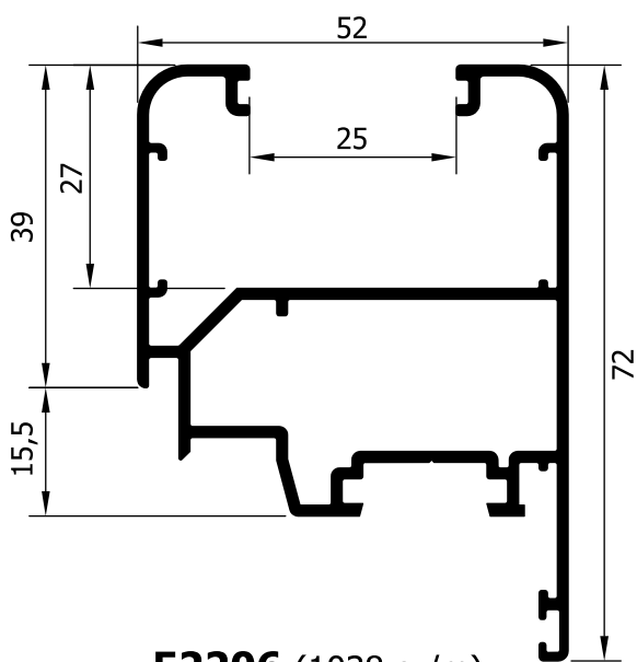
52206 (1038 gr/m) ΦΥΛΛΟ ΚΑΜΠΥΛΟ ΧΩΡΙΣ ΠΗΧΑΚΙ ROUND WING WITHOUT GLASSBEAD
