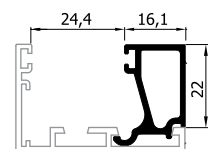
22504 (336gr/m) ΙΣΙΟ ΠΗΧΑΚΙ ΑΣΦΑΛΕΙΑΣ SQUARE GLAZING SAFETY BEAD
