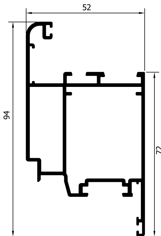
52213 (1321 gr/m) ΦΥΛΛΟ ΚΑΜΠΥΛΟ ΓΙΑ ΠΟΡΤΑ ΧΩΡΙΣ ΤΑΜΠΛΑ ROUND WING FOR DOOR WITHOUT TRANSOM
