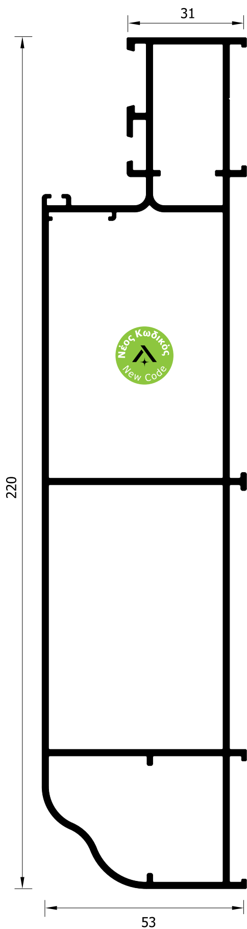
52136 (3185 gr/m) ΚΑΣΑ ΠΑΡΑΔΟΣΙΑΚΗ 220mm TRADITIONAL FRAME 220mm
