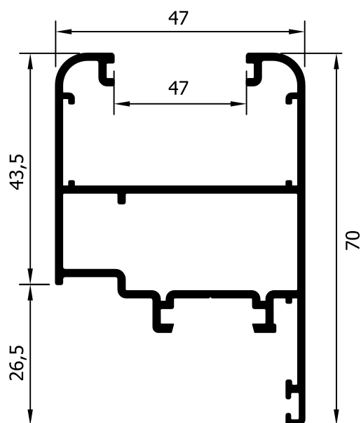
52208 (941 gr/m) ΦΥΛΛΟ ΓΙΑ ΠΑΤΖΟΥΡΙ WING FOR SHUTTER
