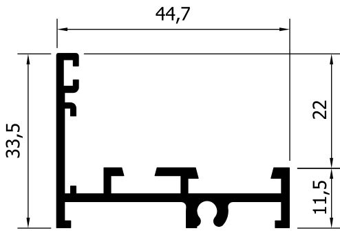
52105 (535 gr/m) ΚΑΣΑ ΙΣΙΑ FLAT FRAME
