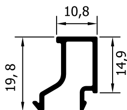
52323 (170 gr/m) ΠΗΧΑΚΙ ΓΙΑ ΚΑΙΤΙΑ 52321, 52322 GLASSBEAD FOR 52321, 52322 (ΓΙΑ ΤΖΑΜΙ ΕΩΣ FOR GLASS UP TO: 16mm)
