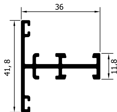
52322 (554 gr/m) ΧΩΡΙΣΜΑ ΓΙΑ ΚΑΙΤΙ ΜΕ ΠΗΧΑΚΙ (σύνδεσμος E - 8221) PARTITION FOR DIVIDER WITH BEAD
