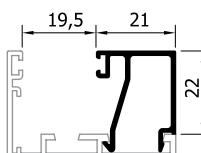
22121 (277 gr/m) ΙΣΙΟ ΠΗΧΑΚΙ SQUARE GLAZING BEAD
