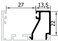
22500 (249 gr/m) ΙΣΙΟ ΠΗΧΑΚΙ SQUARE GLAZING BEAD
