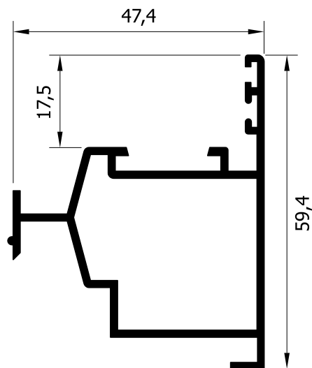
52210 (731 gr/m) ΜΠΙΝΙ ΠΕΡΙΣΤΡΕΦΟΜΕΝΟ ADAPTOR FOR PIVOT WINDOWS
